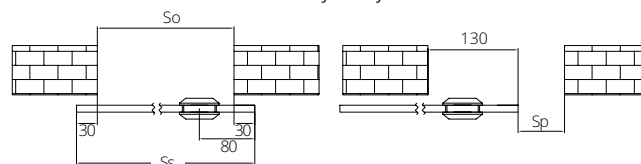
Dvere s diskovým úchytom
