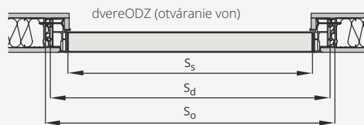
DVERE OTVÁRAVÉ VON ODZ
