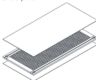
KONŠTRUKCIA KRÍDLA
