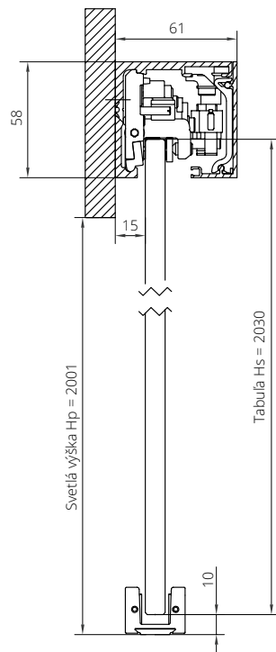
Dvere s podhlovastým úchytom
