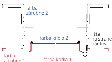
krídlo dvojfarebné / zárubňa dvojfarebná
