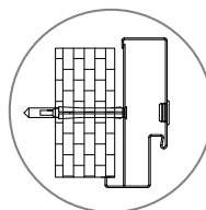
montážny otvor kotva v strede profilu zárubne
