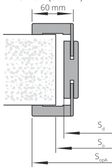
Tunel ZN s obložkou verzia A (60 mm)
