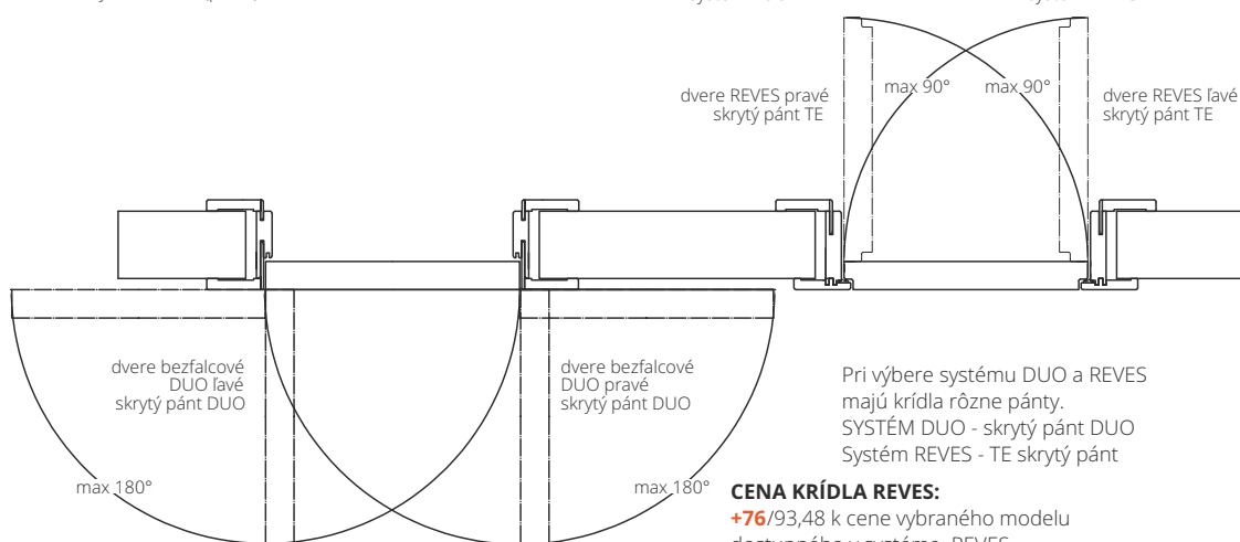
skrytý pánt DUO, strieborná farba - systém DUO
