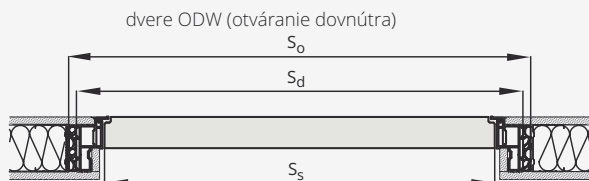
DVERE OTVÁRAVÉ DOVNÚTRA ODW
