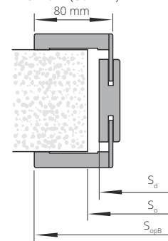
Tunel ZN s obložkou verzia B (80 mm)
